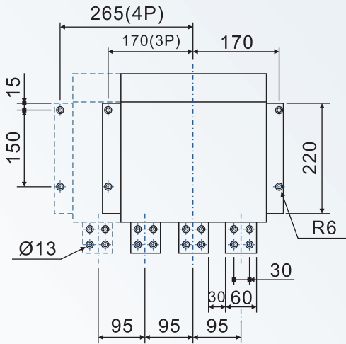
BA2000-H固定式門框(選購)
