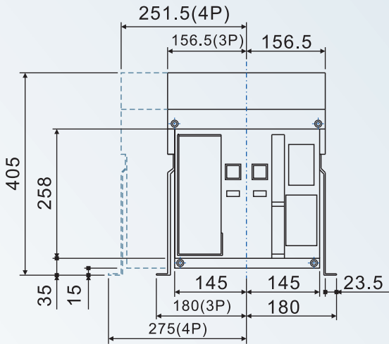
(1) BA2000-H固定式
