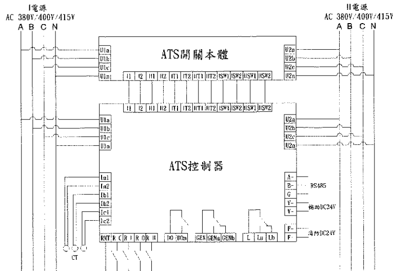
三相四線 380V/400V/415V 系統
