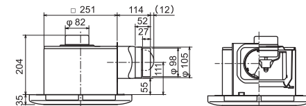
■ 外型圖 (單位:mm)
