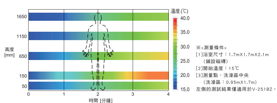
浴室內不同離地高度的溫度變化
