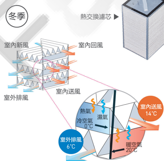
■ 熱交換濾芯內部 (示意機型：FY-15ZY1W)
