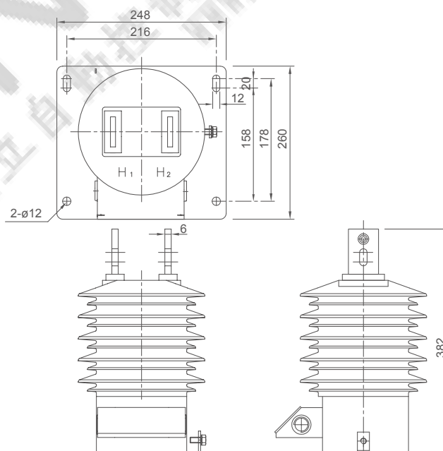
FIG.2 CM-24T
