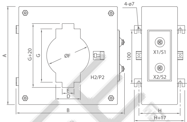
FIG.2 CA-P6, CA-P8
