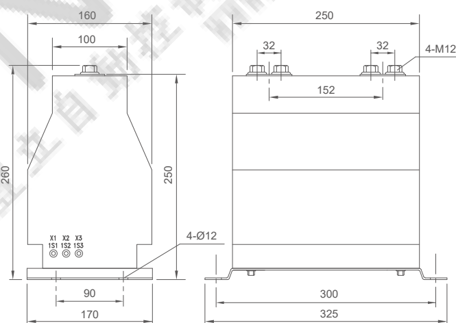
FIG.1 CM-6FV
