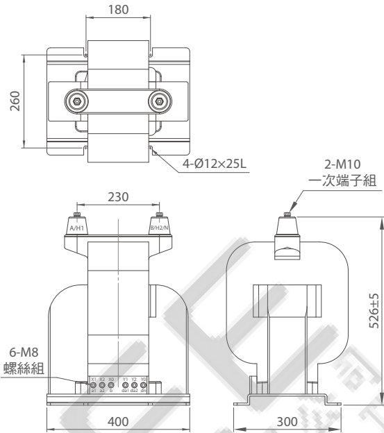
FIG.1 TM-2TF
