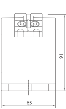
FIG.1 CA-PVA
