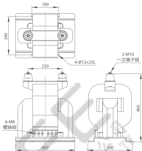
FIG.1 TM-2HF
