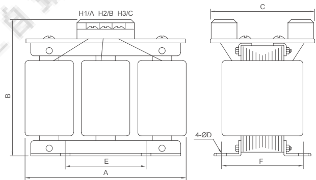
FIG.2 3Ø, TR
