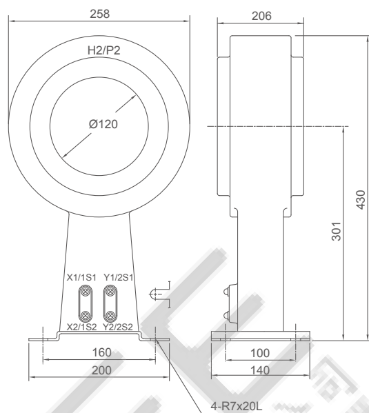
FIG.1 CGD-2MV
