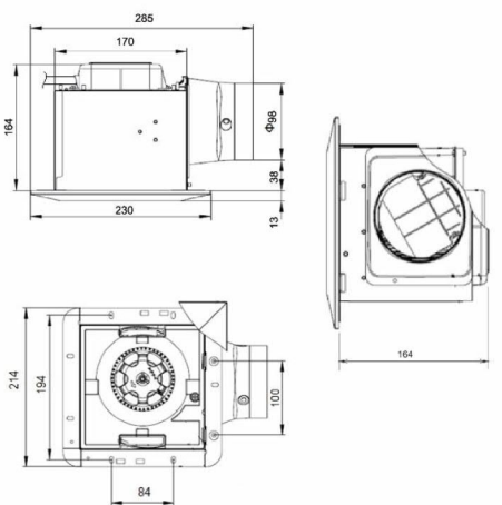
FV-17CU8R / FV-17CU8W 設計·施工用圖 單位: mm (毫米)
