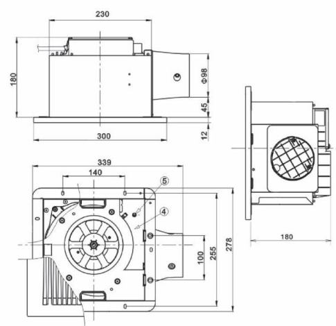
FV-24JR2W 設計-施工用圖
