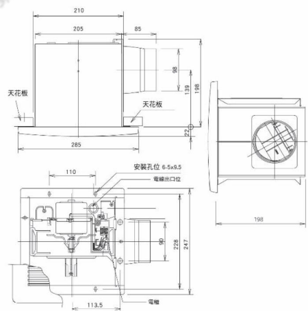
FV-21CV2R / FV-21CV2W 設計·施工用圖 單位: mm (毫米)
