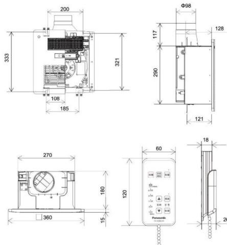
FV-30BU3R / FV-30BU3W 設計·施工用圖 單位: mm (毫米)
