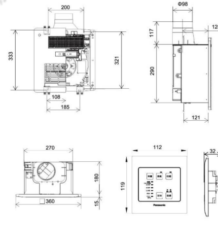
FV-30BUY3R / FV-30BUY3W 設計·施工用圖 單位: mm (毫米)
