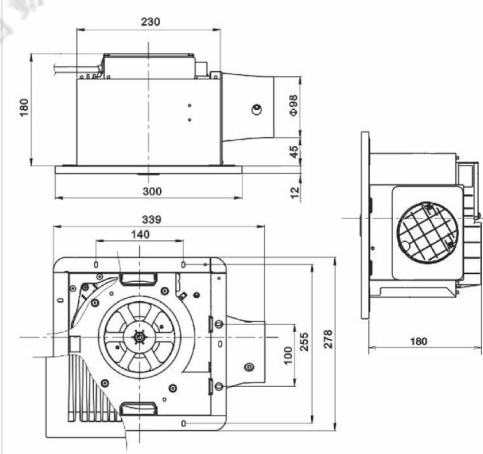
FV-24JA2W 設計-施工用圖
