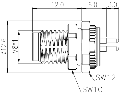
公端插座
