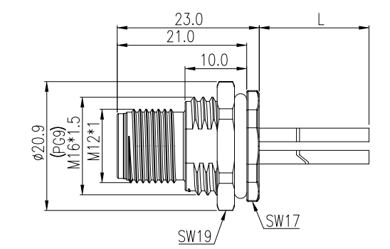
公端插座
