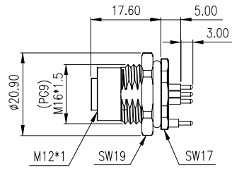
母端插座
