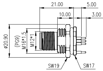
公端插座
