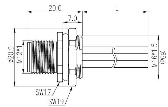
公端插座
