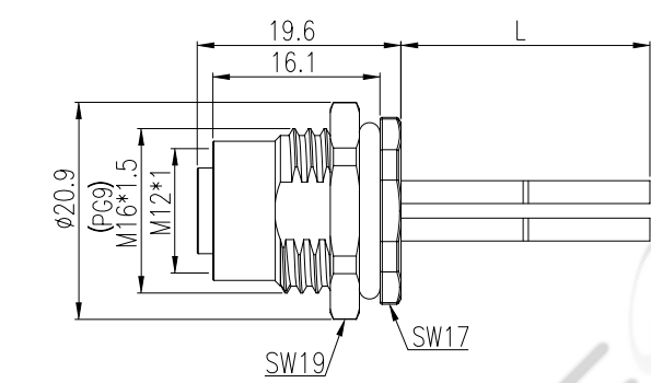
母端插座
