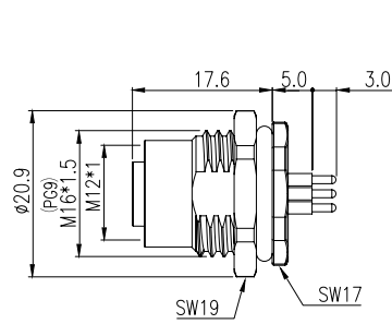
母端插座
