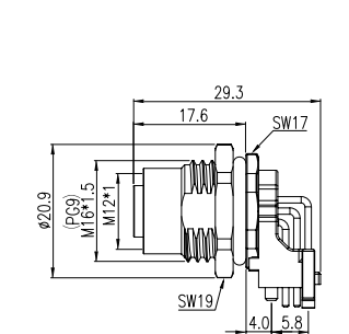
母端插座
