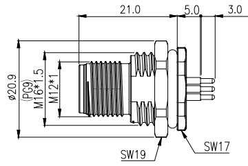
公端插座
