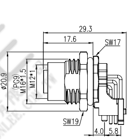
母端插座
