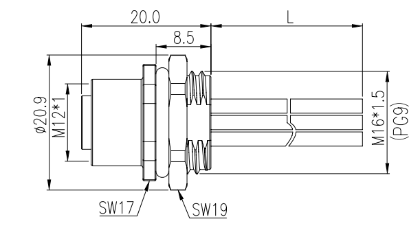
母端插座
