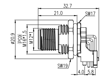
公端插座
