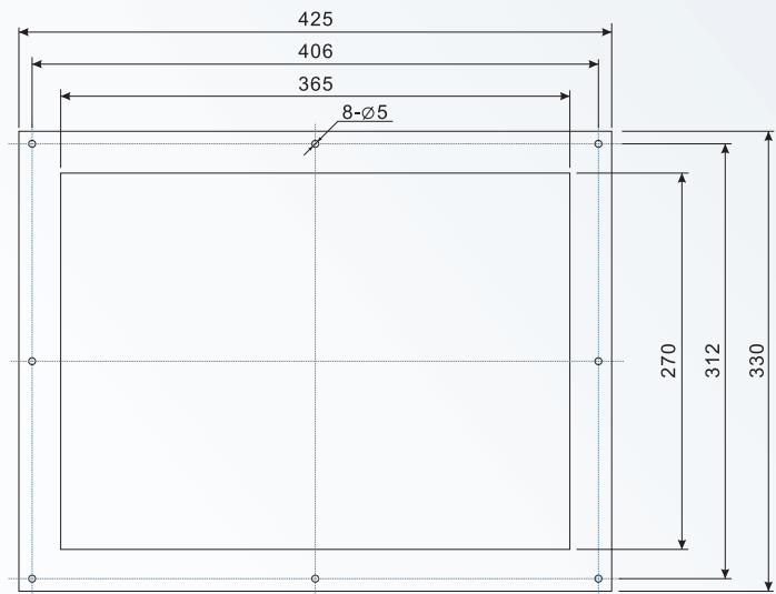
BA3200-H固定式門框(選購)
