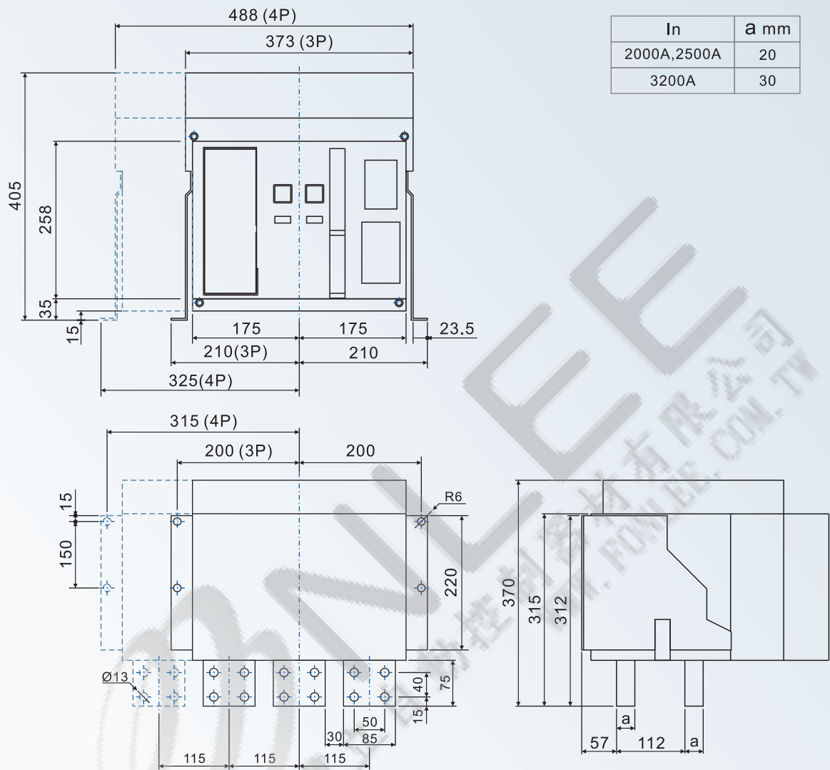
BA3200-H固定式門框(選購)
