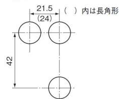
トランス付の 最小取付ピッチ
