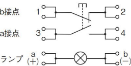
回路図
