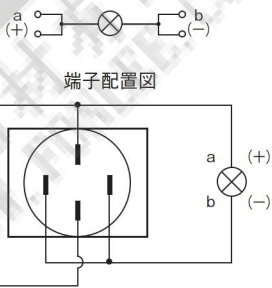
回路図
