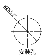
安裝孔尺寸圖
