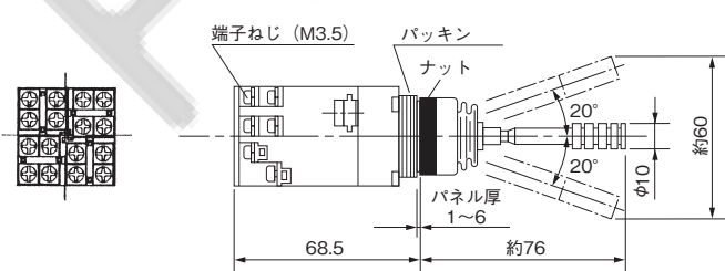
〈はんだ兼タブ端子／AR22A2H・A7H形〉
