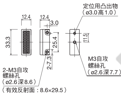
IAC-R7M 型 (背面 / 側面安裝)
