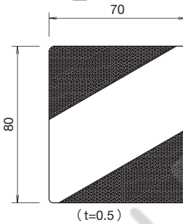
IAC-R7B 型 (背面安裝)
