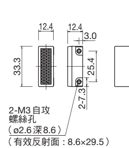
IAC-R7S 型 (側面安裝)
