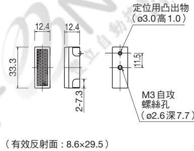
IAC-R7B 型 (背面安裝)
