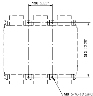
开孔图
