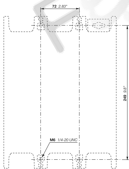
开孔图
