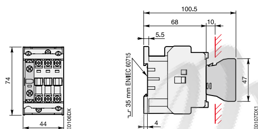
NX + CA5X前装1极辅助触点模块
