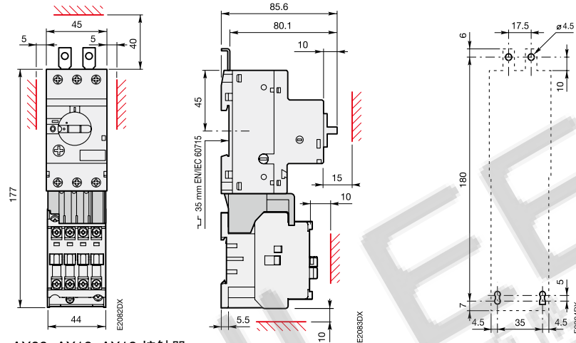
AX09, AX12, AX18 接触器 + BEA 16/116 + MS 116
