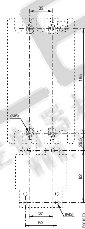
开孔图
