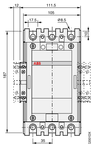
AX185, AX205 c/w 1 x CAL18X + VM 300H 机械联锁
