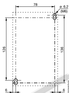
开孔图
