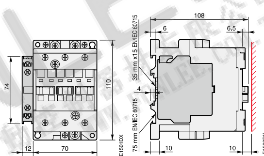
+ CAL5X侧装2极辅助触点模块
