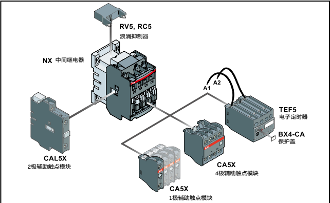
附件装配图（其它附件也可提供）
