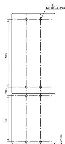
开孔图
