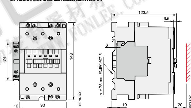
AX95, AX115, AX150 + CAL18X侧装2极辅助触点模块
