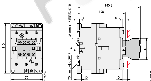
+ CA5X前装4极辅助触点模块及相对的2层结构
