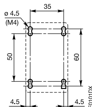
开孔图
