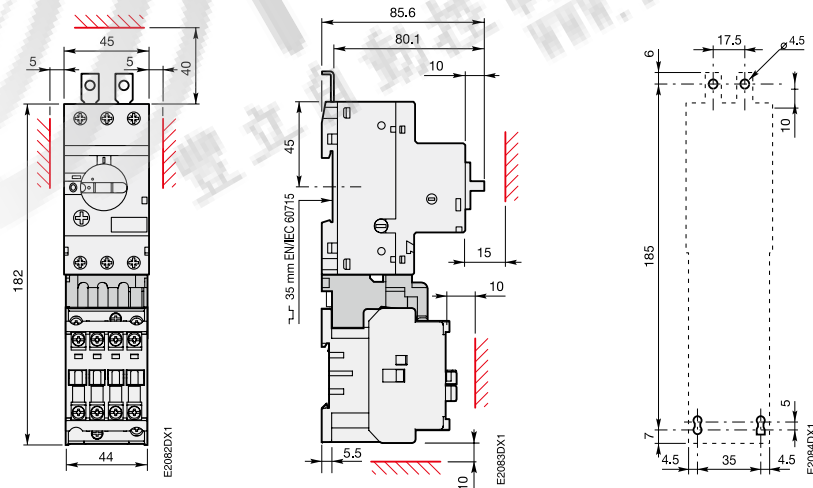
AX25 接触器 + BEA 25/116 + MS 116
