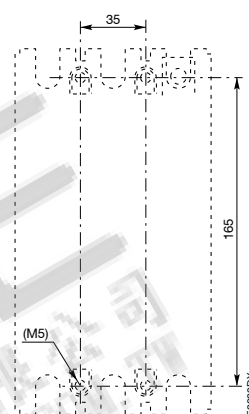
开孔图
