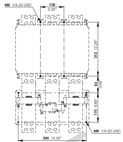
开孔图
