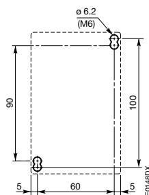
开孔图
