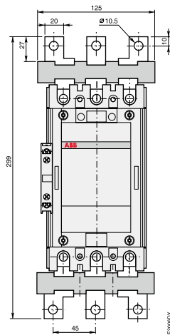
AX185, AX205 c/w 1 x CAL18X + LW 185 扩展端子
