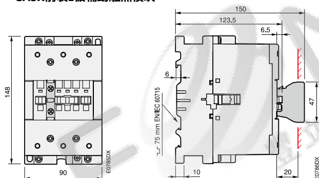
AX95, AX115, AX150 + CA5X前装1极辅助触点模块
