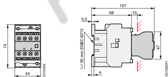
NX + TEF 5 前装电子定时器
