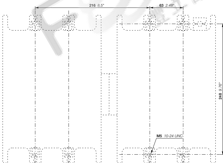
开孔图
