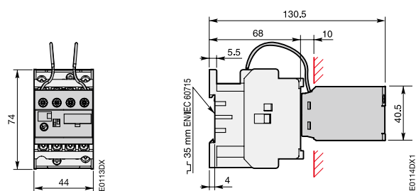
NX + TEF 5 前装电子定时器
