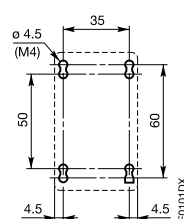
开孔图
