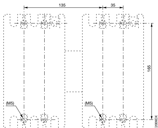
开孔图
