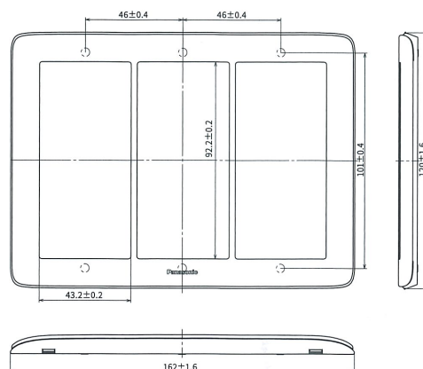
開關係列用蓋板 (3連用)
