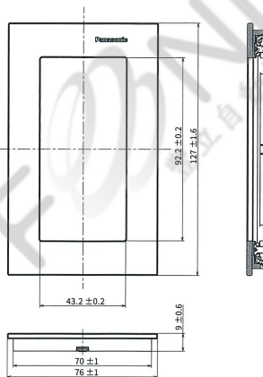
玻璃蓋板 (1連用)
