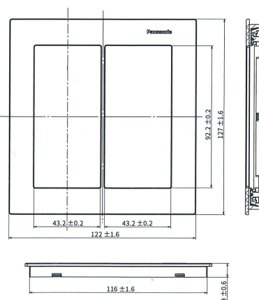
鋁合金 / 不鏽鋼蓋板 (2連用)
