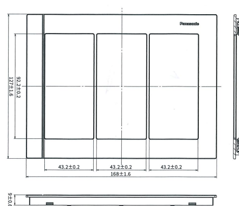
鋁合金蓋板 (3連用)
