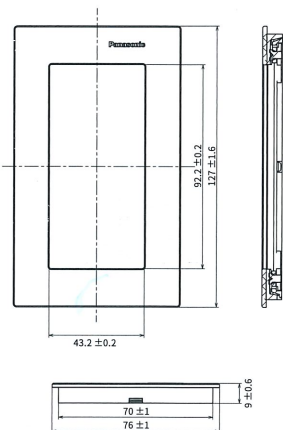
鋁合金 / 不鏽鋼蓋板 (1連用)
