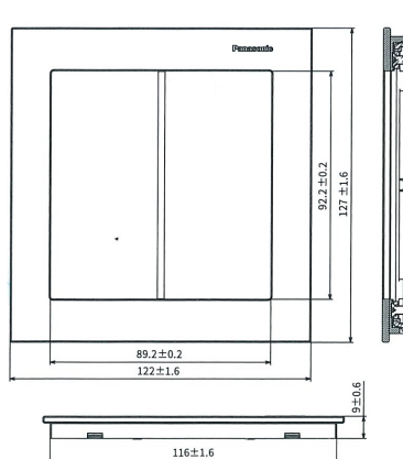
玻璃蓋板 (2連用)
