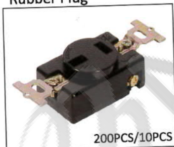
WJ-1220 電木暗插座 Receptacle
