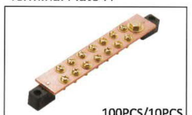
WJ-9114 動力端子板 14P Power Grounding Terminal Plate 14P
