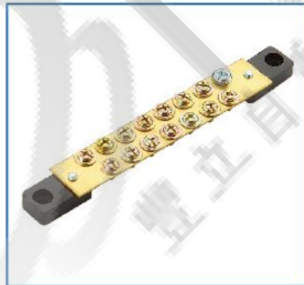
WJ-9014 接地端子板 14P Grounding Terminal Plate
