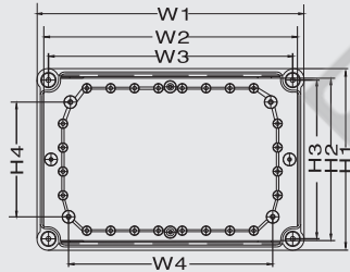
Dimension(允许误差 ± 1mm)
