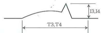
(註二)閉路, 開路控制電流時間特性
