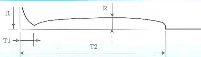
(註一)閉路操作電流時間特性
