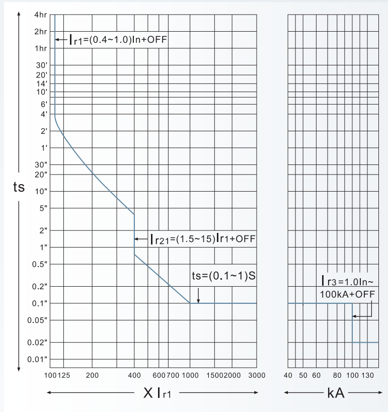
c.III 極動作曲線 (BA4000-H、BA5000-H、BA6300-H)
