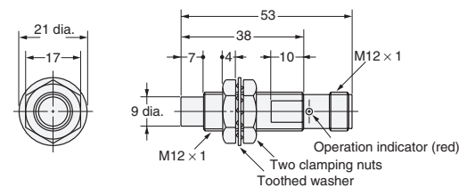
Diagram 19 E2E-X5MY□-M1
