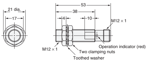
Diagram 18 E2E-X2Y□-M1
