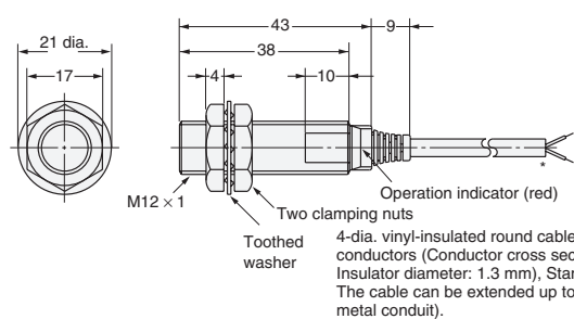
Diagram 7 E2E-X2Y□
