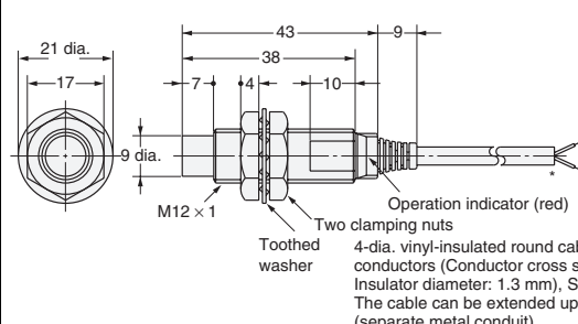
Diagram 8 E2E-X5MY□
