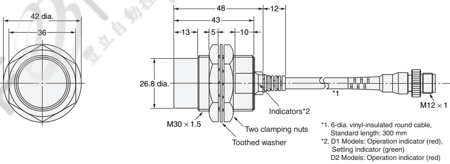
Diagram 33 E2E-X20MD1-M1GJ E2E-X20MD1-M1TGJ E2E-X20MD□-M1TGJ-US
