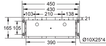
4P-100A及225A 以下(高啟斷)型式
