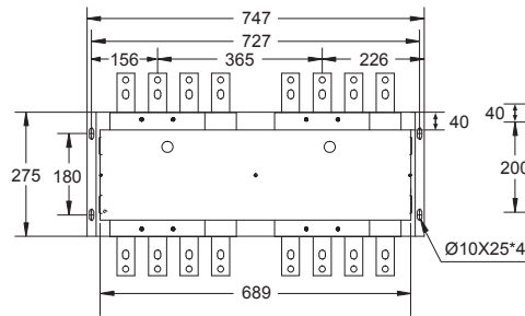
4P-600~800A 以下型式
